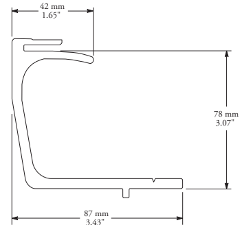
1. 40RF006455601 Matl: PVC
