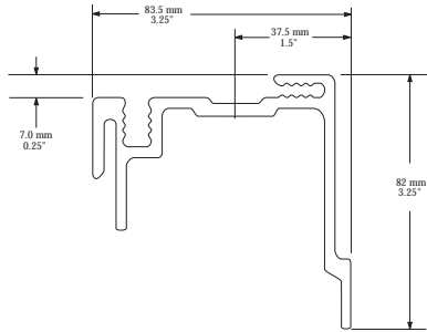
1. 39RFDF1398 Matl: PVC
